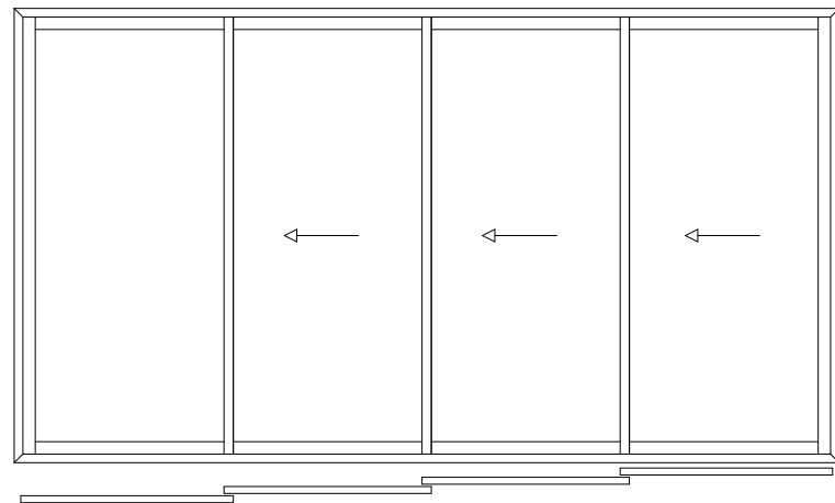
4 RAIL UITVOERING: XOOO
